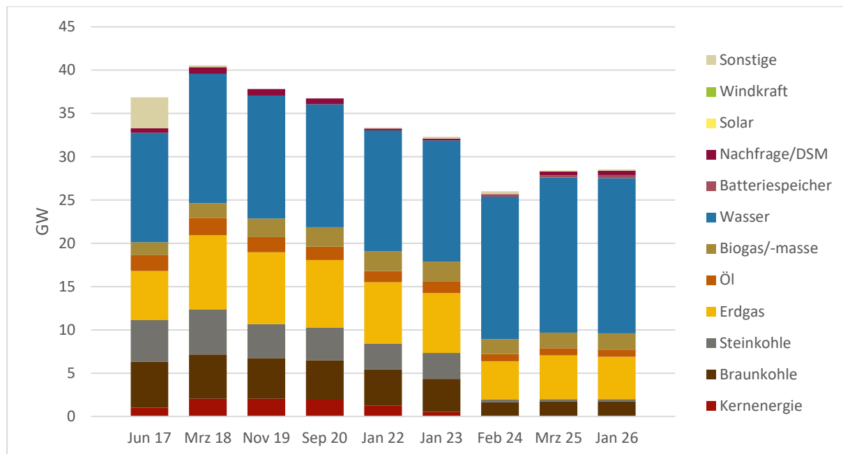
Abbildung 4: Präqualifizierte positive mFRR (in GW) je Primärenergieträger/Kategorie in Deutschland
