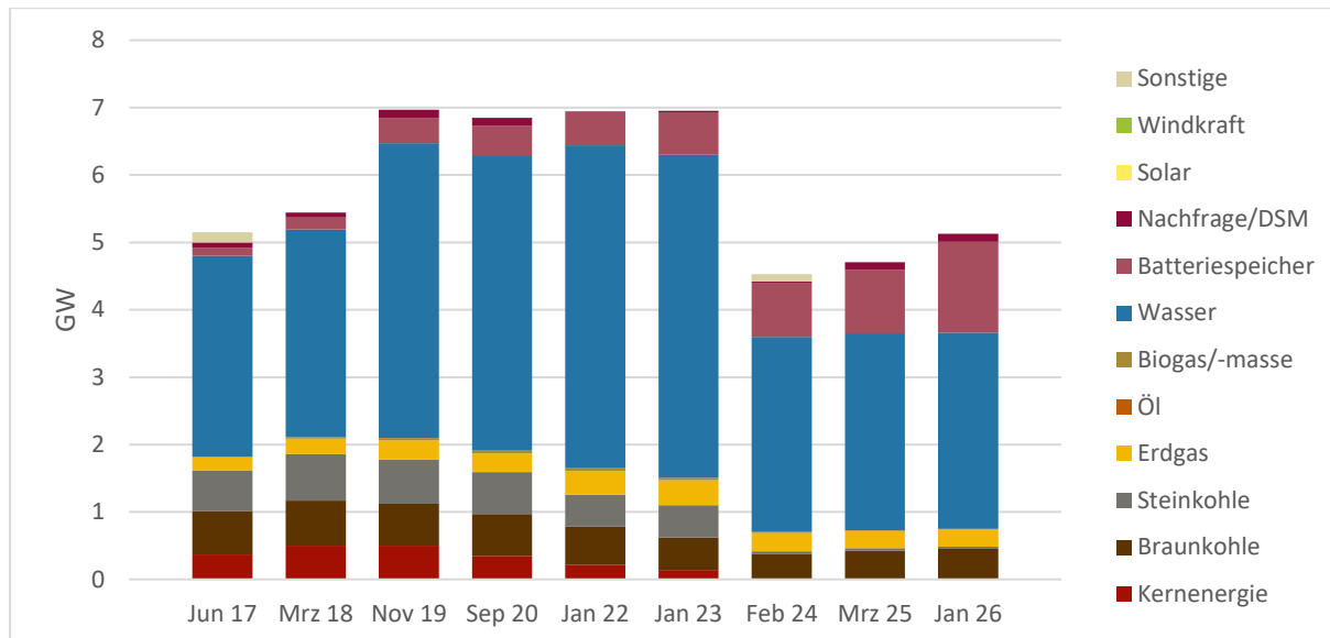
Abbildung 1: Präqualifizierte FCR (in GW) je Primärenergieträger/Kategorie in Deutschland
