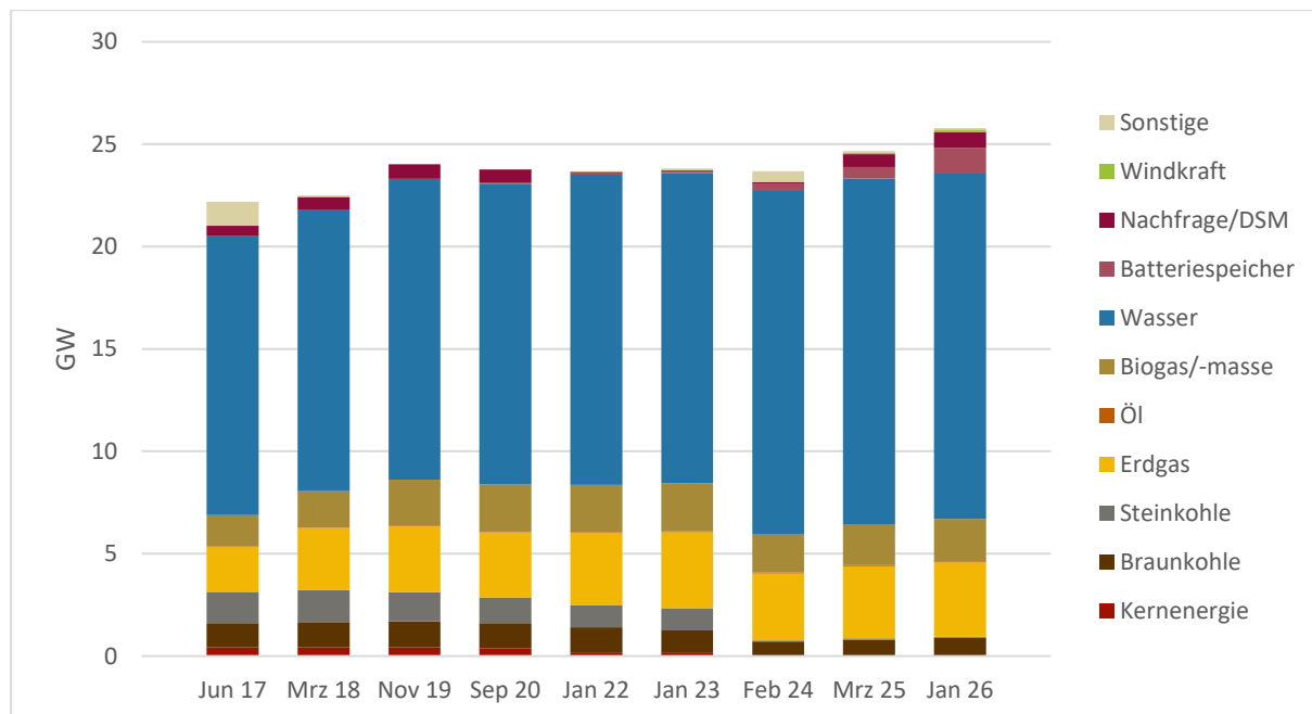
Abbildung 3: Präqualifizierte negative aFRR (in GW) je Primärenergieträger/Kategorie in Deutschland
