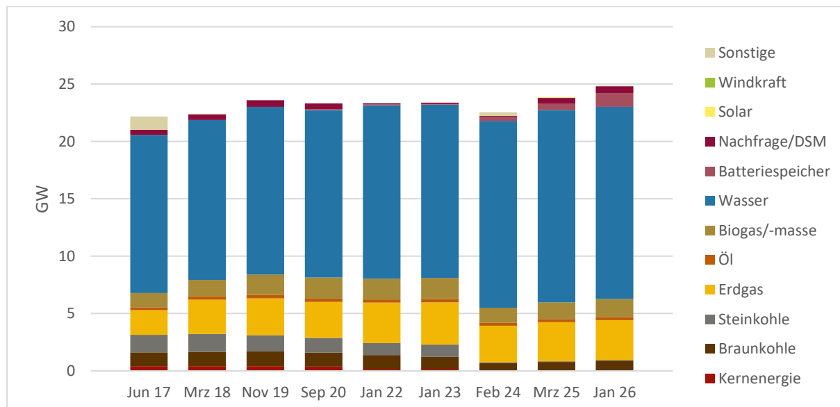
Abbildung 2: Präqualifizierte positive aFRR (in GW) je Primärenergieträger/Kategorie in Deutschland
